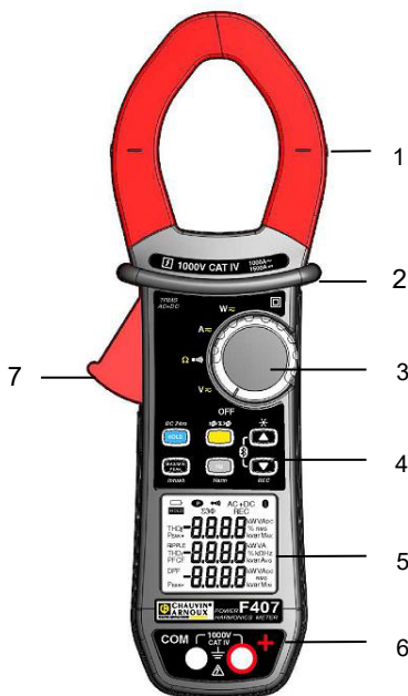
Figuur 1: de multimetertang F407
