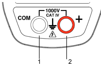
Figuur 5: de klemmen
