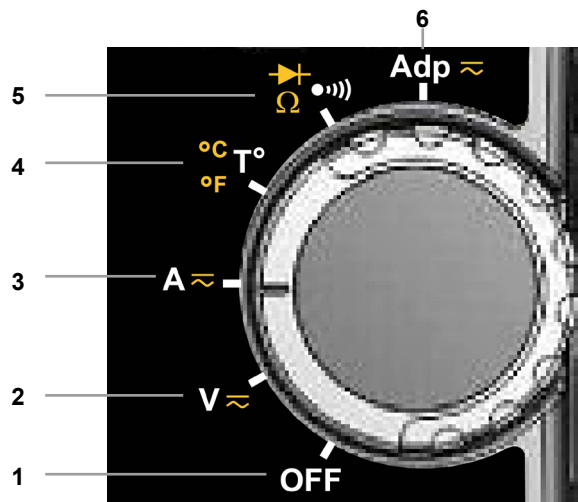
Figure 2 : Le commutateur
