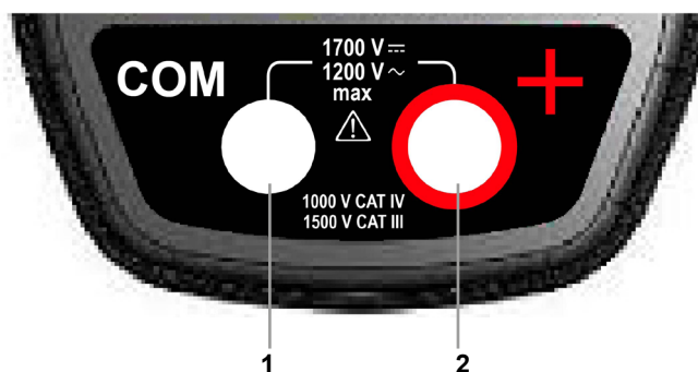
Figure 5 : Les bornes
