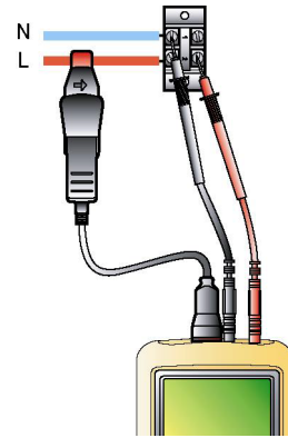
Figura 74: Connessione in monofase. 005
