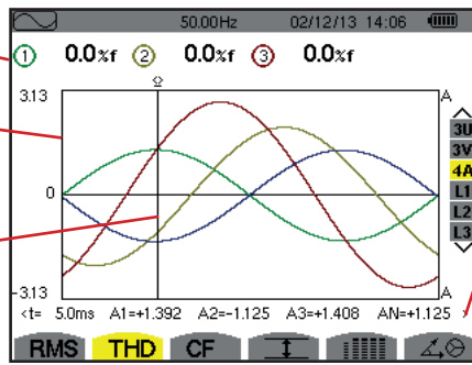
Figura 59: La pantalla de visualización THD en 4A
