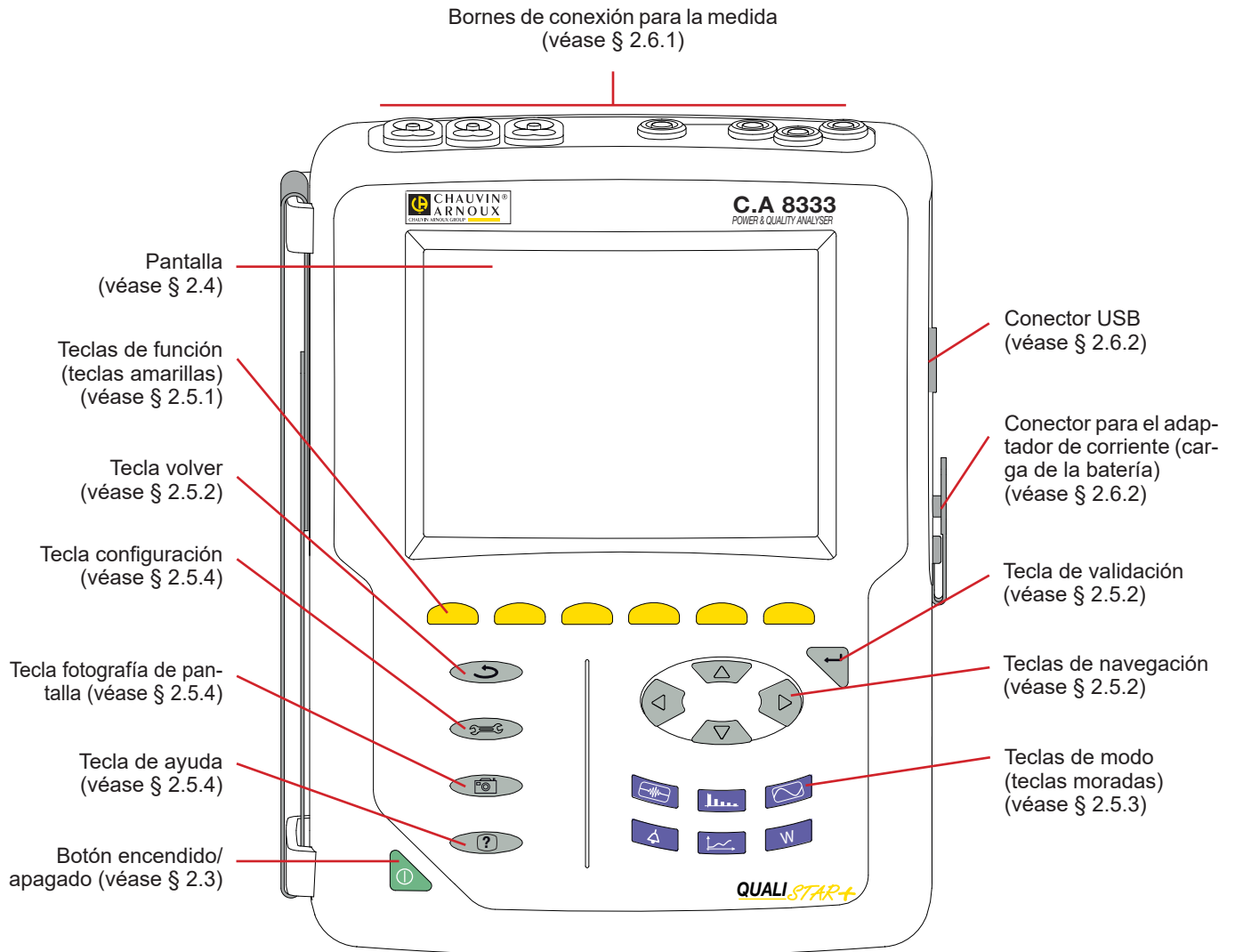
Figura 2: Vista general del Qualistar+
