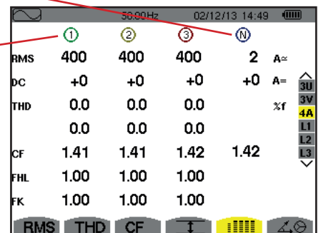
Figura 69: La pantalla de visualización simultánea en 4A
