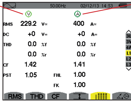
Figura 70: La pantalla de visualización simultánea en L1
