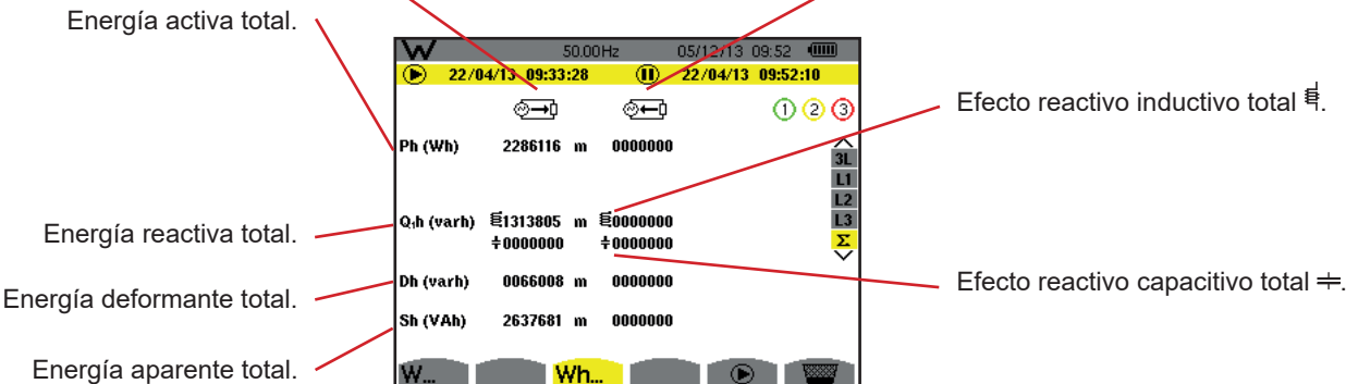
Figura 104: La pantalla de visualización de las energías consumidas y aportadas totales en Σ
