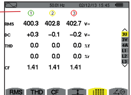
Figura 67: La pantalla de visualización simultánea en 3U
