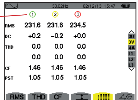
Figura 68: La pantalla de visualización simultánea en 3V
