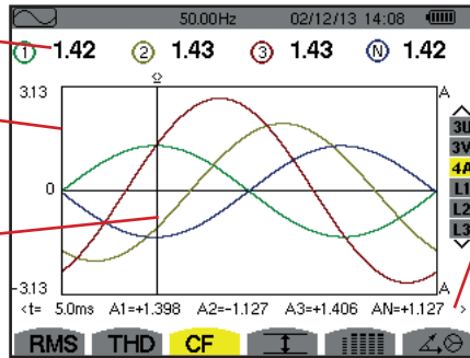
Figura 62: La pantalla de visualización CF en 4A
