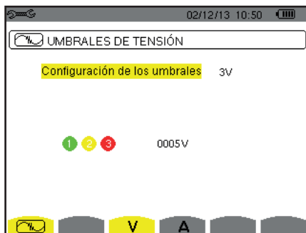
Figura 29: La pantalla Umbrales de tensión en el menú Modo transitorio
