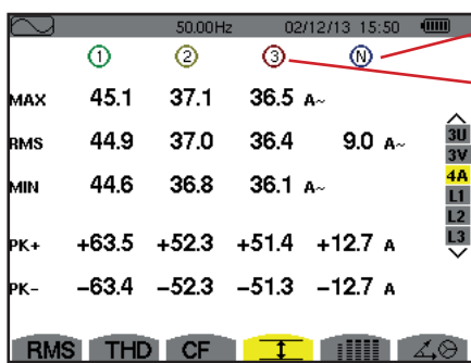
Figura 65: La pantalla de visualización Máx.-Mín. en 4A
