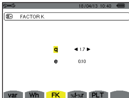
Figura 23: El menú Selección de los coeficientes de cálculo del factor K
