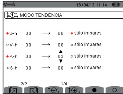
Figura 33: La segunda pantalla del Modo tendencia que se está modificando
