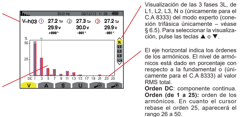
Figura 42: Ejemplo de visualización de los armónicos de la tensión de fase en 3L
