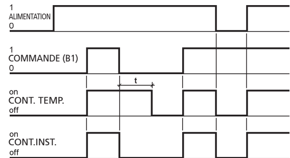
Retard à la retombée RDT.x2c-x8c
