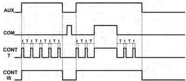
F5 – Clignoteur, asymétrique.
