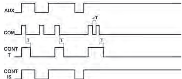
F1 – Temporisation à la retombée, les contacts instantanés suivent l'état de l'alimentation auxiliaire.
