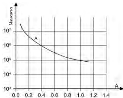
Charge du contact : 110 Vdc, L/R 40 ms
