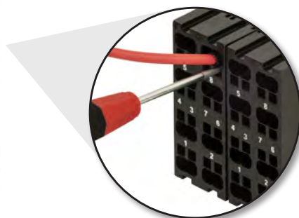
Détail des connexions
