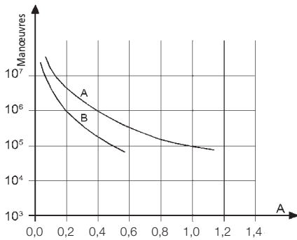
Charge sur le contact : 110 Vdc, L/R 40 ms Courbe A : RMM.x6-7-8 Courbe B : RMM.x2-3-4
