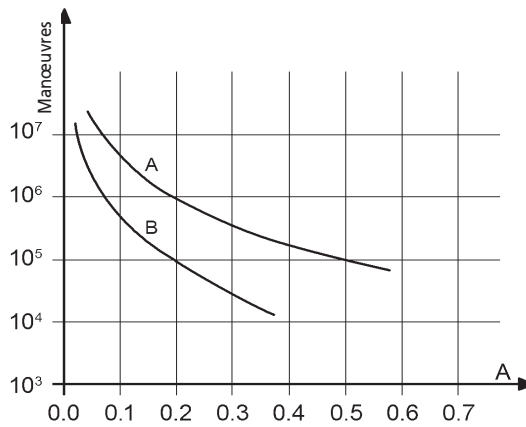
Charge sur le contact : 110 Vdc, L/R 40 ms Courbe A : RDT_x7-x8-x9 Courbe B : RDT_x1-x2-x4
