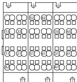
PRIR242 Modèle avec numérotation pour RVLV16/2
