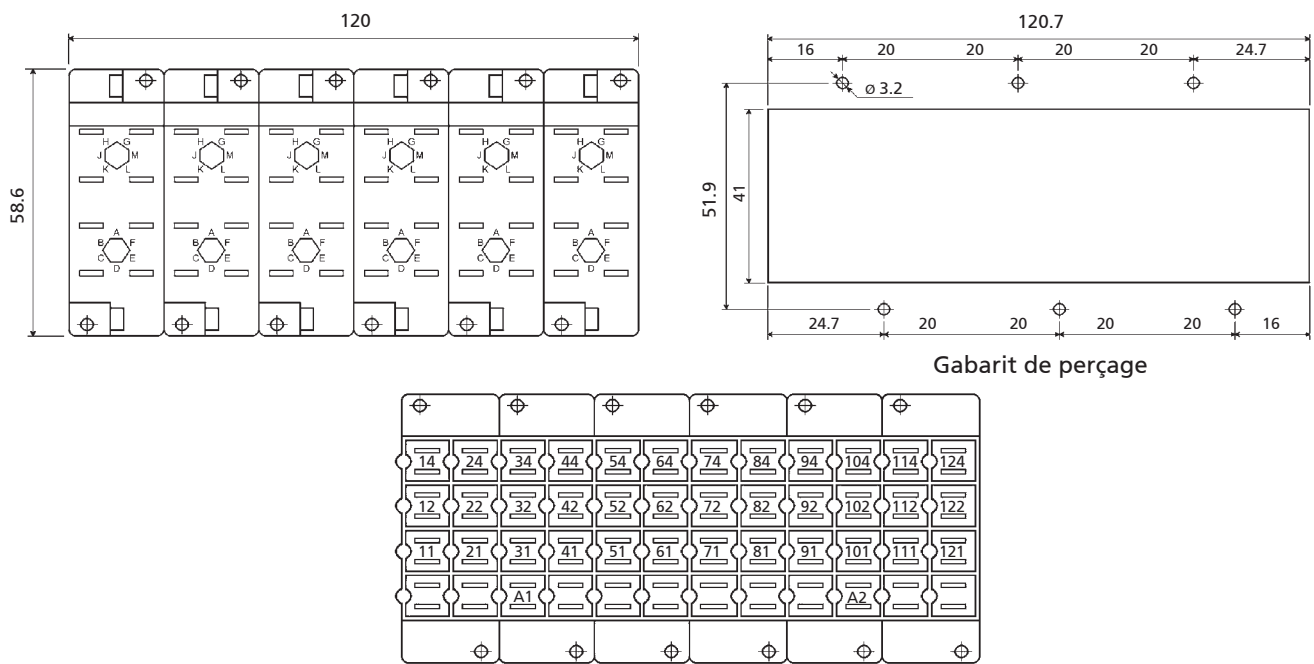
ADF6-ESAPOK / Modèle avec numérotation "ESAPOK"
