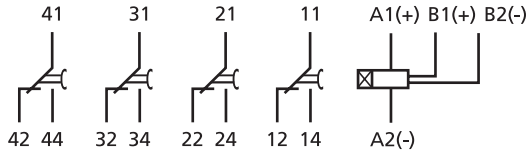
Schéma "appel" RDT.x4c-x9c
