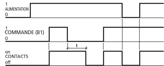
Retard à la retombée RDT.x1c-x7c
