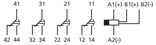
Schéma "retombée" RDT.x4c-x9c
