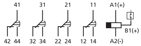
Schéma "retombée" RDT.x1c-x7c
