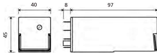
Relais avec réglage par vis fendue à tête plate
