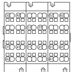
PRIR244 Modèle avec numérotation pour RVLV16/5
