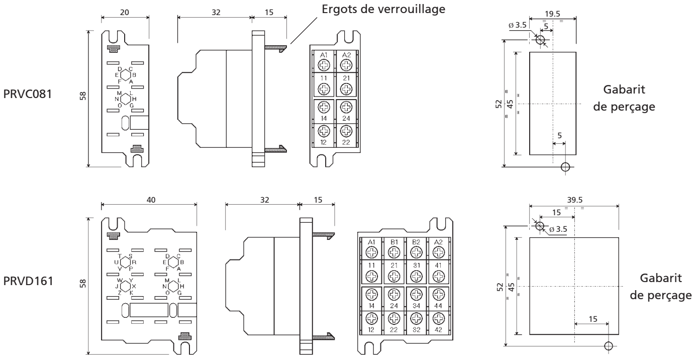
Détail des raccordements
