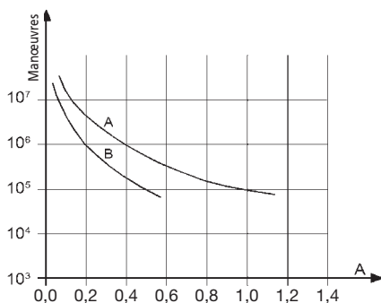
Charge sur le contact : 110 Vdc, L/R 40 ms Courbe A : RGM.x7 Courbe B : RGM.x3-4-5 (sans contact NO/NF)
