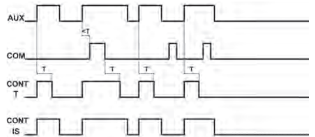
F3 – Fonction passage.
