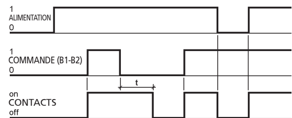
Retard à la retombée RDT.x4c-x9c
