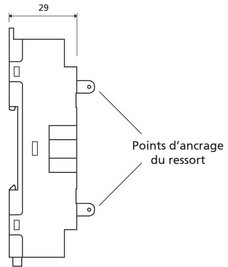
Vue latérale
