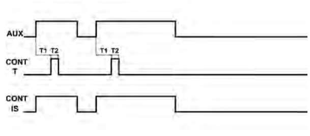
F7 – Fonction passage avec impulsion fixe (3 s), retardée à l'appel.
