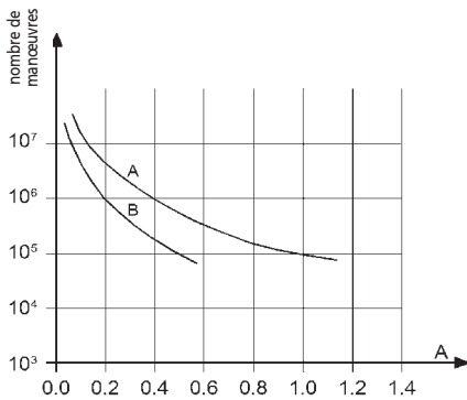
Charge sur le contact : 110 Vdc, L/R 40 ms Courbe A : RMM.x6X Courbe B : RMM.x2X
