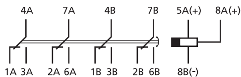
Temporisation à la retombée
